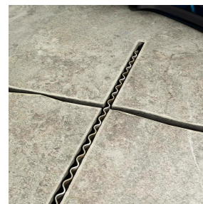
2. Insérer les joints ondulés.
