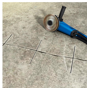
1. Élargir les flancs des fissures et fraisier en croix tous les 15 - 20 cm.
